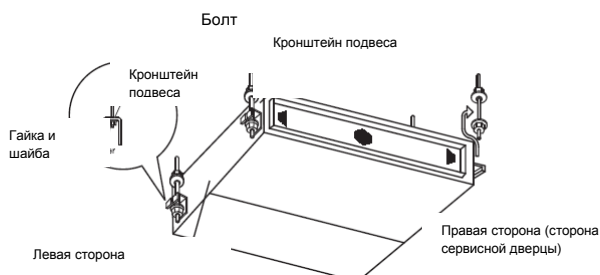
Рис. 4.6. Подвес внутреннего блока
