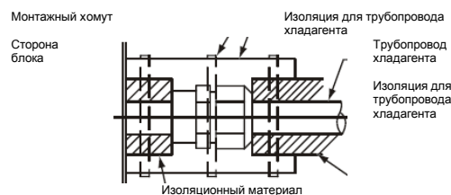
Рис. 5.3. Изоляция трубопровода.
