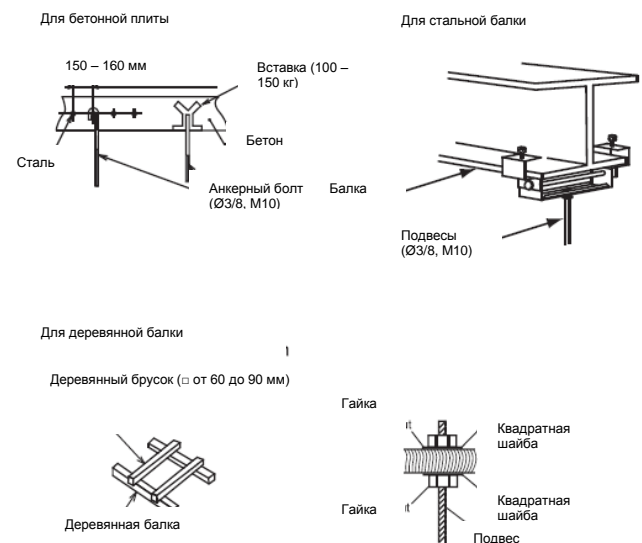
Рис. 4.2 Монтаж подвесов
