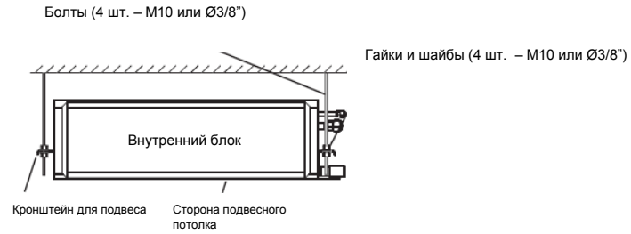
Рис. 4.4 Подвес внутреннего блока
