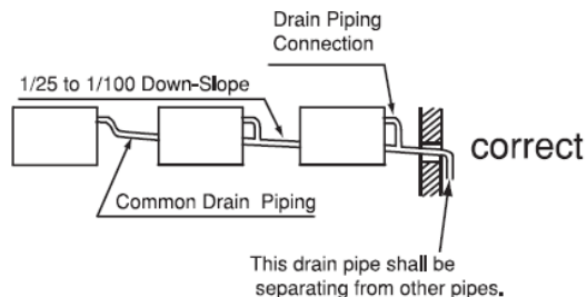
Рис. 6.1. Сливной трубопровод
