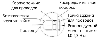
Деталь «R» в увеличенном виде (схема затяжки зажима для проводов)
