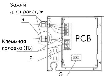
Схема расположения клемм электродвигателя
