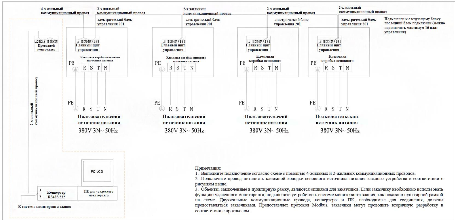
(4) Принципиальная схема соединений устройств
